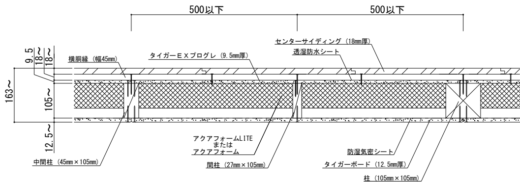
水平断面図
